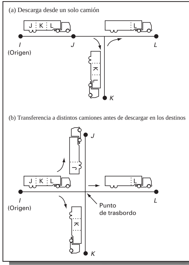
Figura 6-10 Ejemplos del privilegio de parada para descarga parcial.
