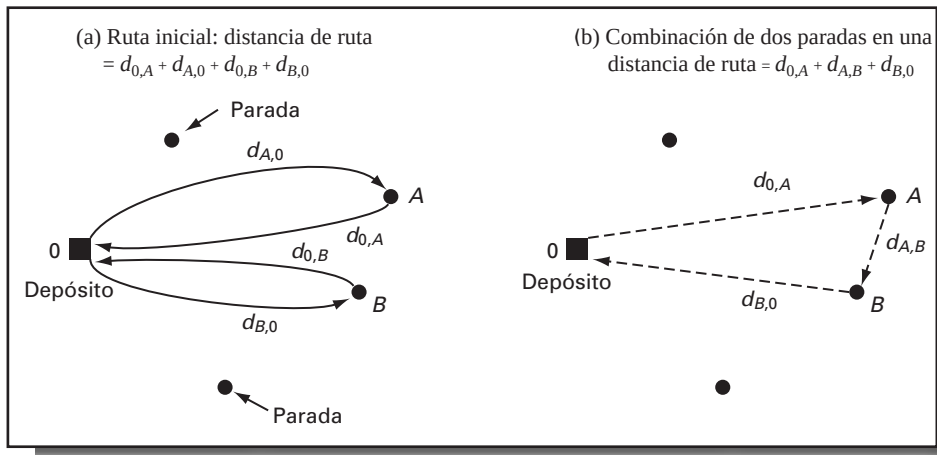
Figura 7-15 Distancia reducida de viaje mediante consolidación de paradas en una ruta.
